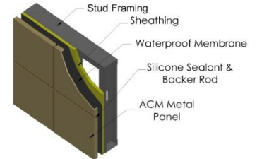
GN-2000
